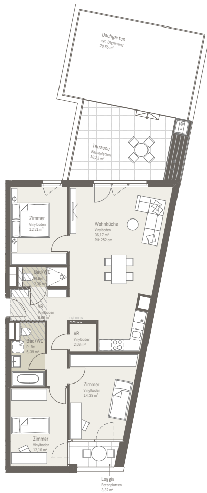
TOP30 Maßstab 1:200
