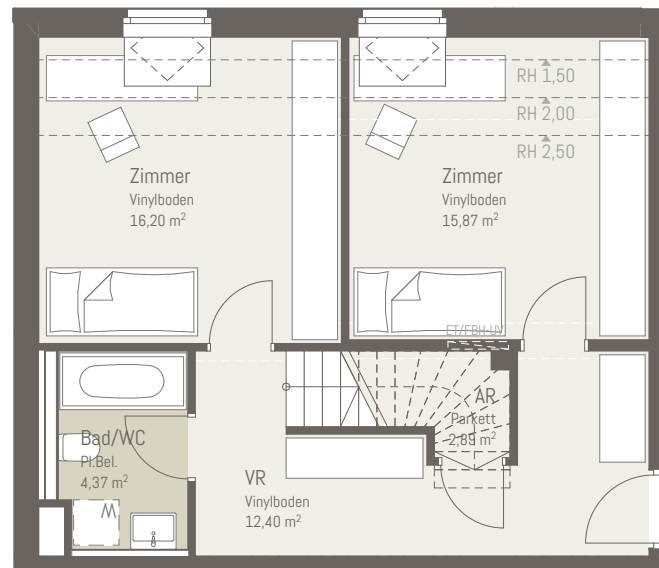
1. Dachgeschoß
