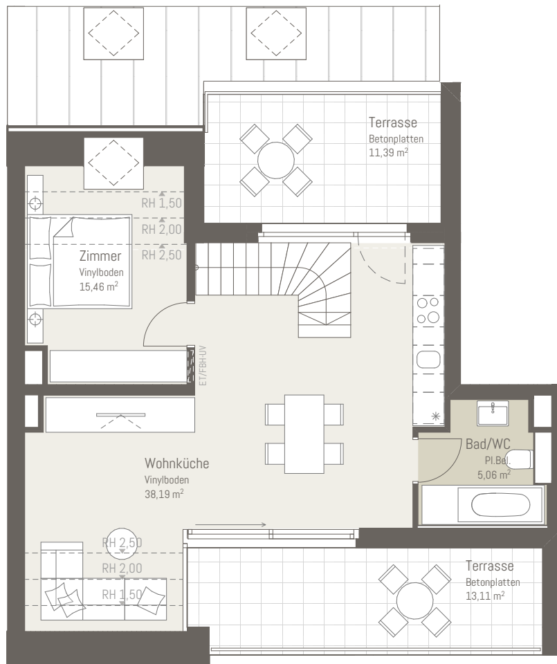
2. Dachgeschoß
